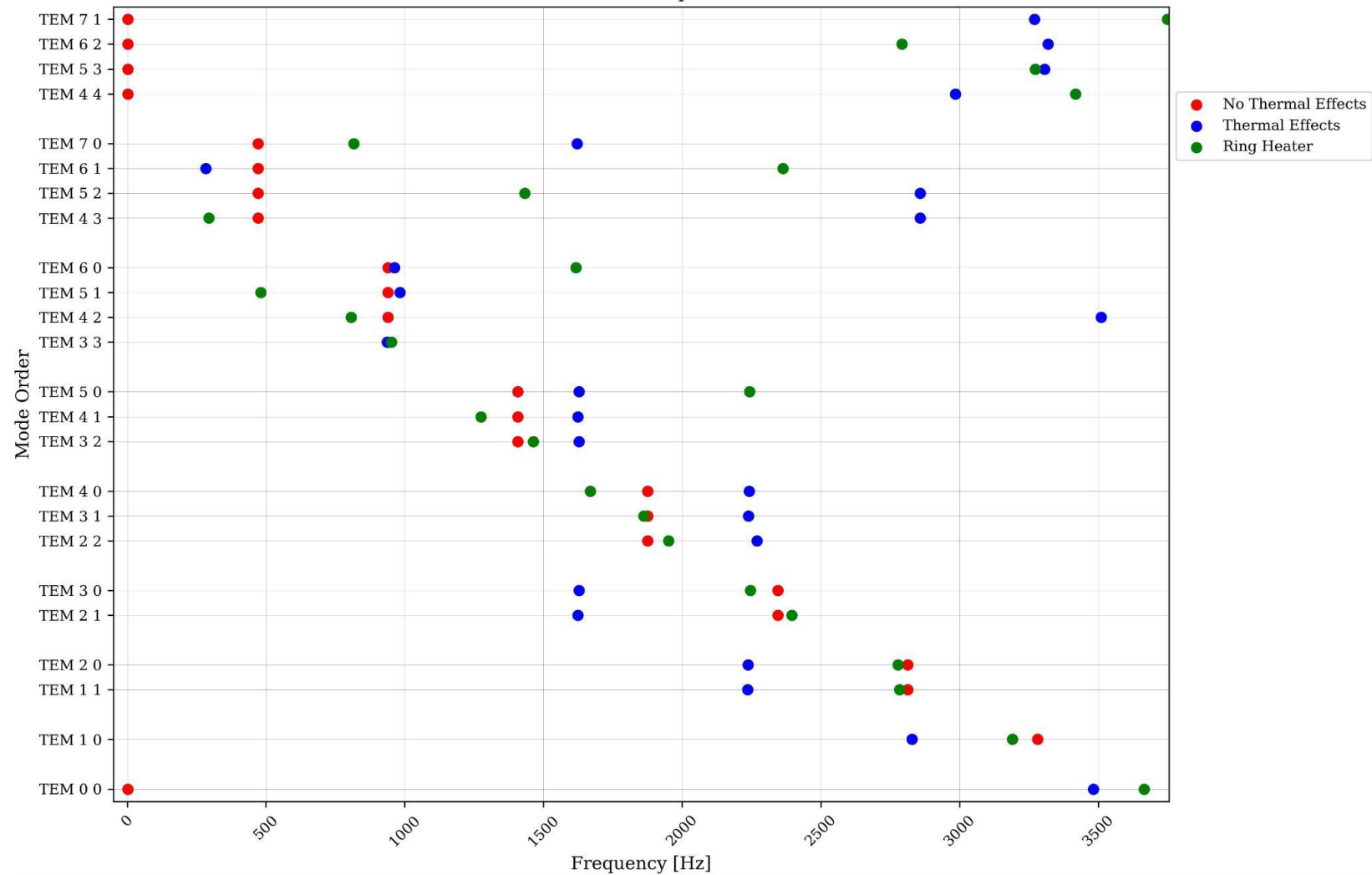
TEM Mode Frequencies
