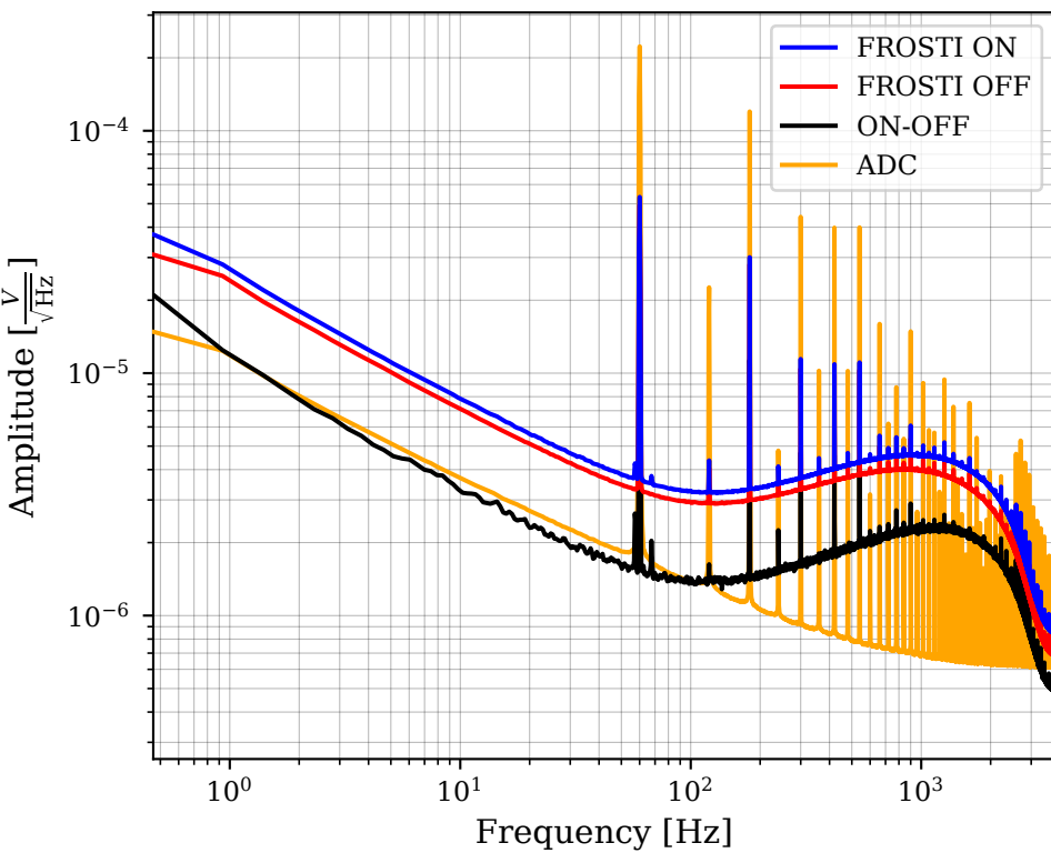
CH0 ASDs
